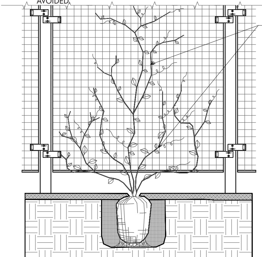
ELEVATION
